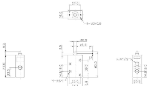
Zawór 3 drogowy 2 położeniowy z rolką Przyłącze - 1/8
