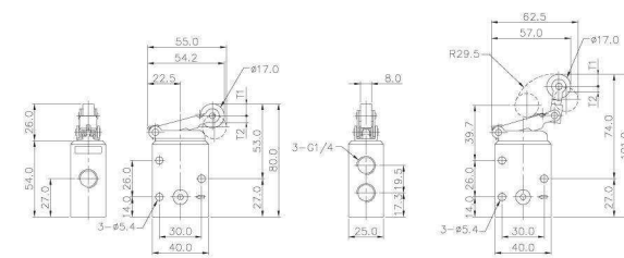
Zawór 3 drogowy 2 położeniowy sterowany bezpośrednio (przełącznik) Przyłącze - 1/4
