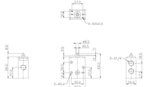
Zawór 3 drogowy 2 położeniowy z rolką Przyłącze - 1/4
