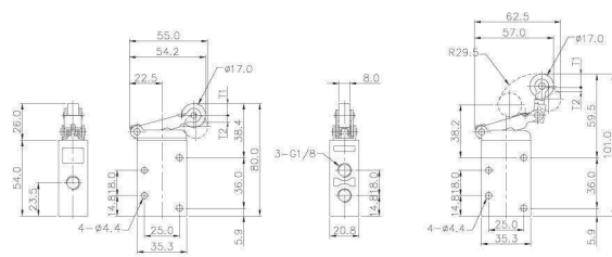
Zawór 3 drogowy 2 położeniowy sterowany bezpośrednio (przełącznik) Przyłącze - 1/8
