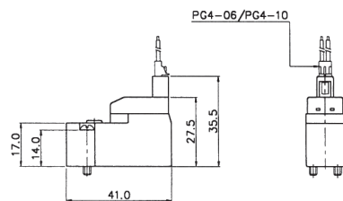
YSV20-DP-SL-**-** Normalnie zamknięty
