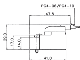
YSV20-DP-SM-**-** Normalnie zamknięty
