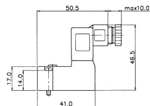
YSV20-DP-SC-CN1-**-** Normalnie zamknięty
